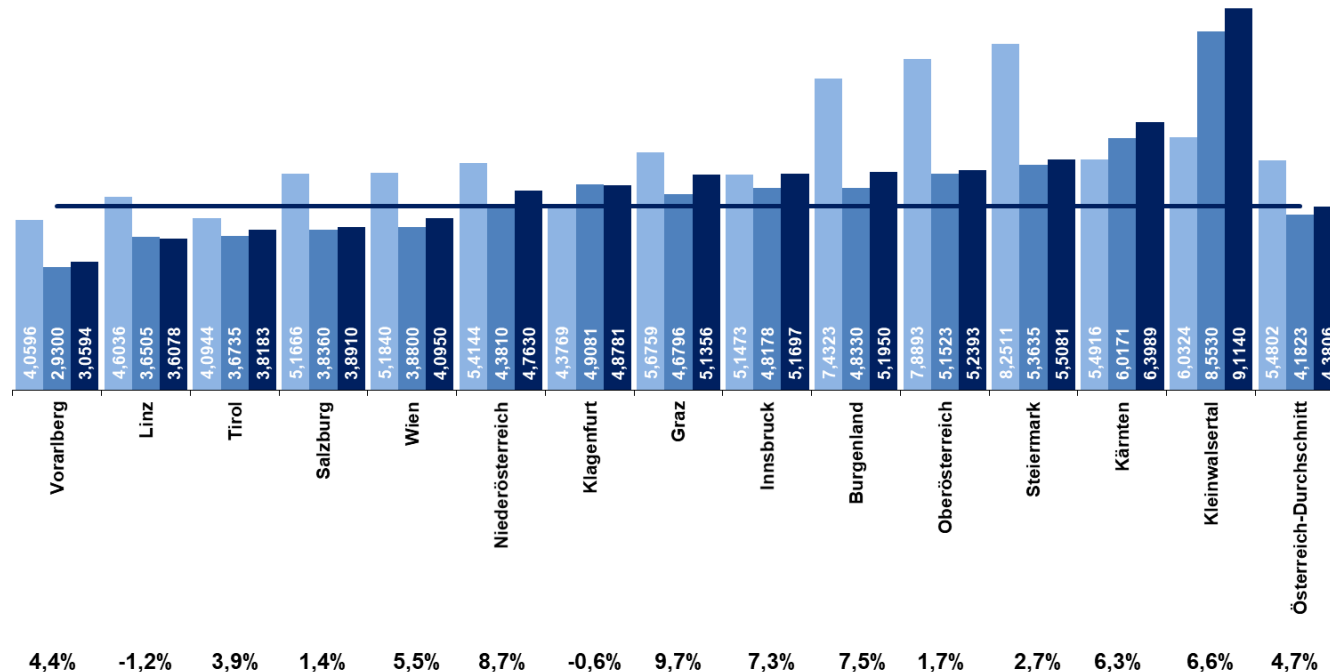
Netznutzungs- und Netzverlustentgelt: Entwicklung zum Vorjahr in % Netzebene 7 gemessen BD = 3.000 h Cent/kWh
