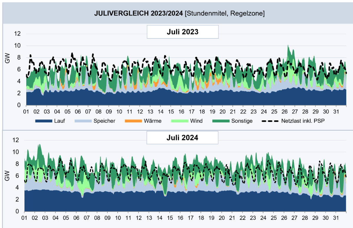
Abbildung 6: Realisierte Bedarfsdeckung Juli 2023 und 2024, Regelzone
