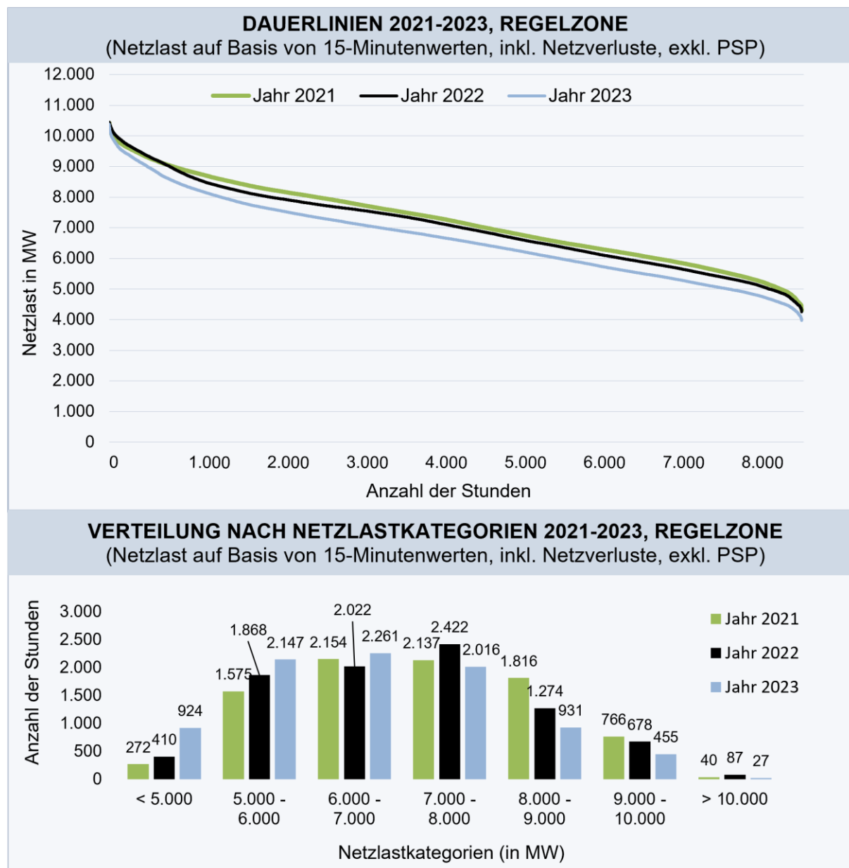
Abbildung 4: Dauerlinien und Verteilung der Netzlast für 2021-2023, Regelzone
