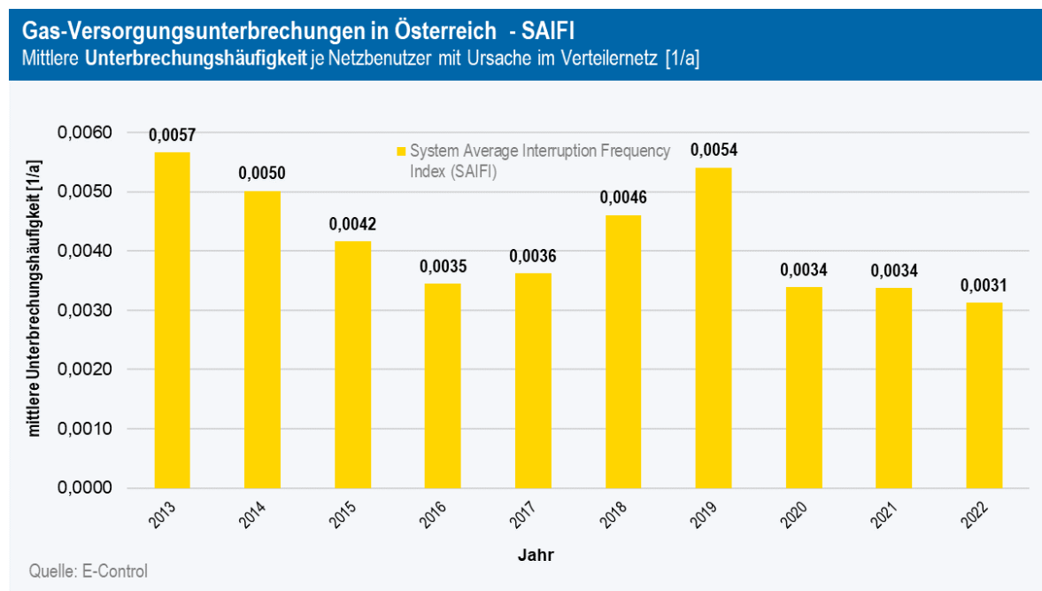
Abbildung 6: Entwicklung SAIFI 2013 bis 2022 für Österreich gesamt
