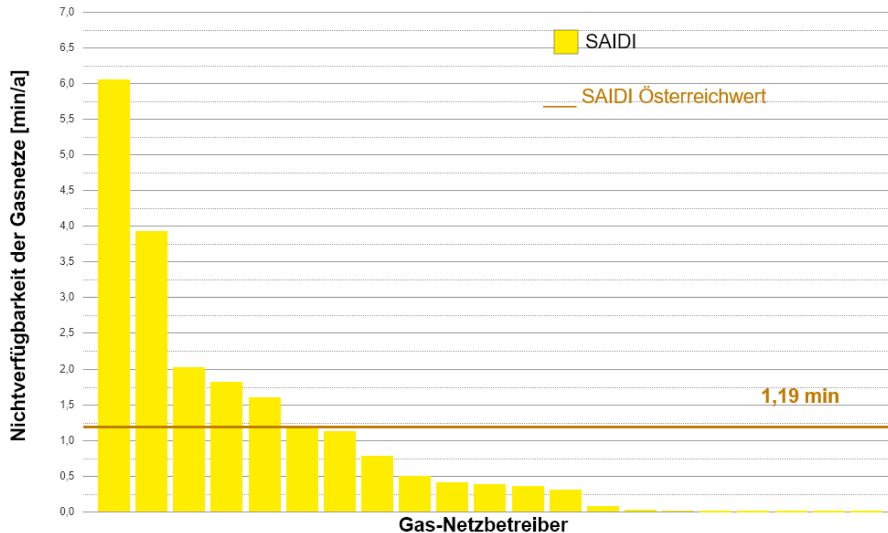
Abbildung 8: SAIDI (System Average Interruption Duration Index) im Jahr 2022, in Minuten/Jahr, je Netzbetreiber sowie durchschnittliche Unterbrechungsdauer je Netznutzer in Österreich
