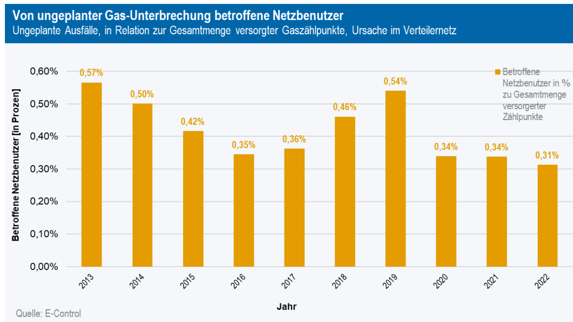
Abbildung 4: Entwicklung von ungeplanter Gas-Unterbrechung betroffene Netzbenutzer mit Ursache im Verteilernetz 2013 bis 2022 [in Prozent]
