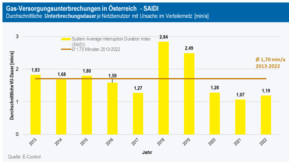
Abbildung 5: Entwicklung SAIDI 2013 bis 2022 für Österreich gesamt
