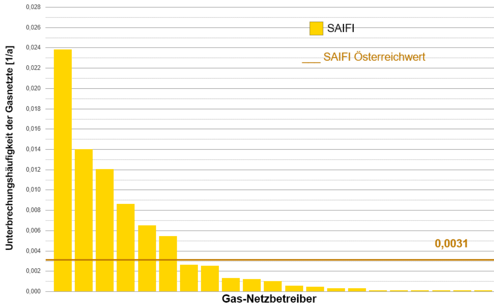
Abbildung 9: SAIFI (System Average Interruption Frequency Index) im Jahr 2022, in 1/Jahr, je Netzbetreiber sowie durchschnittliche Unterbrechungshäufigkeit je Netznutzer in Österreich
