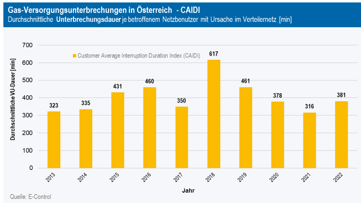
Abbildung 7: Entwicklung CAIDI 2013 bis 2022 für Österreich gesamt
